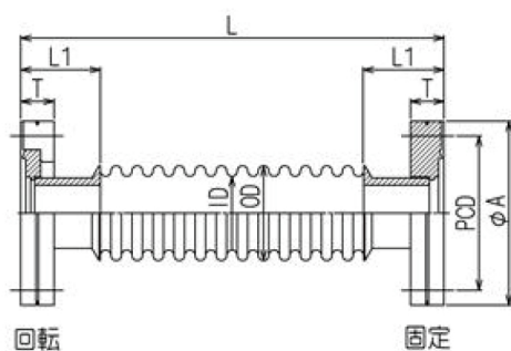
外観寸法図
