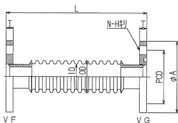
外観寸法図
