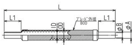
外観寸法図
