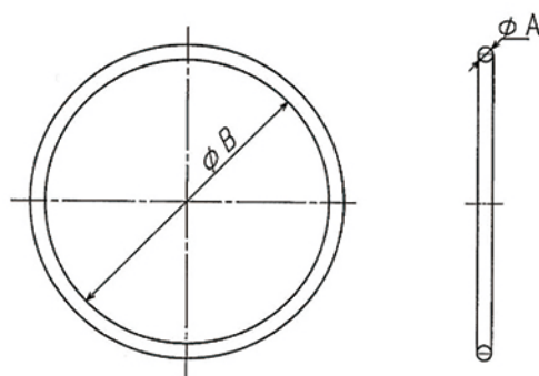
外観寸法図
