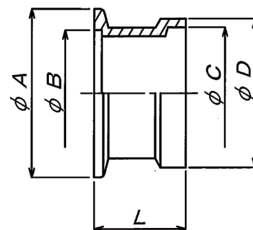
外観寸法図
