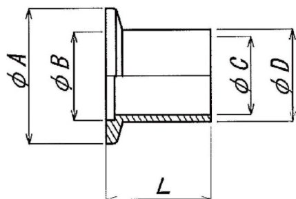
外観寸法図
