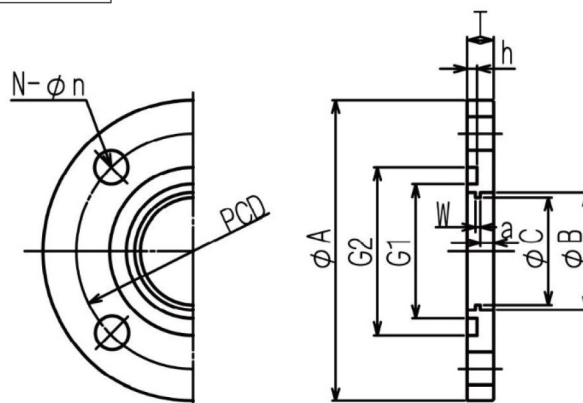
外観寸法図
